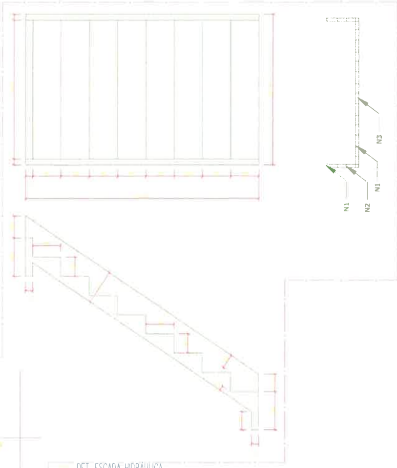
DET. ESCADA HIDRÁULICA ESCALA 1:25
