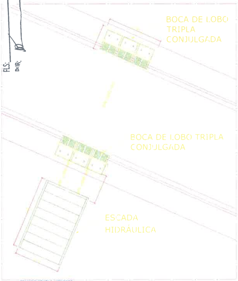
DETALHAMENTO DRENAGEM R. SANTOS DAMINI
