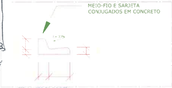
DET. A - MEIO-FIO E SARJETA A04 ESCALA 1:10
