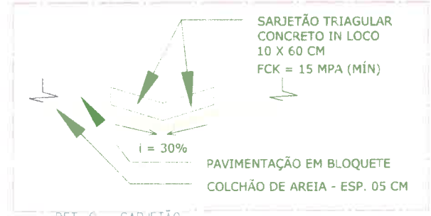
DET. C - SARJETÃO A04 ESCALA 1:10
