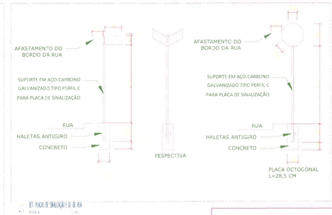
DET. PLACAS DE SINALIZAÇÃO E ID. DE RUA
