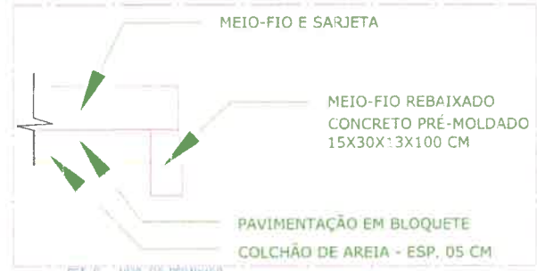
DET. B - MEIO-FIO REBAIXADO A04 ESCALA 1:10
