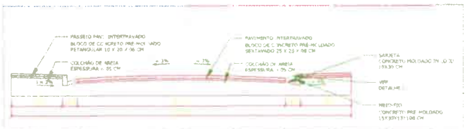
PERFIL R. DO CAMPO E R. SCS DUMONT A04 ESCALA 1:10
