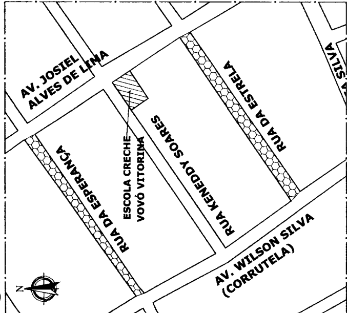
02 IMPLANTAÇÃO MUTIRÃO ESCALA 1:1000
