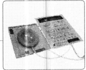
PÁ DE CHOQUE COM SENSOR DE FEEDBACK DE RCP
