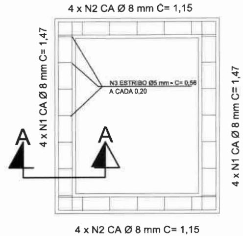
ARMAÇÃO
