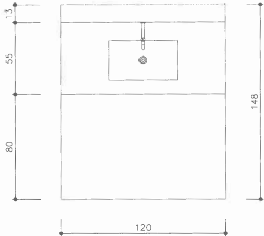
PLANTA BAIXA
