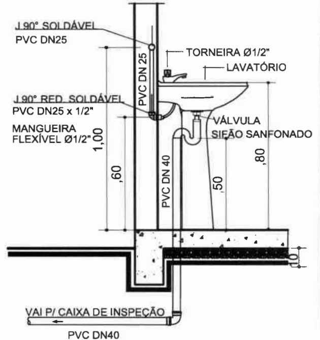
INSTALAÇÃO - LAVATÓRIO
