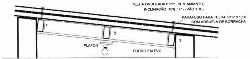
CORTE AA Sem escala
