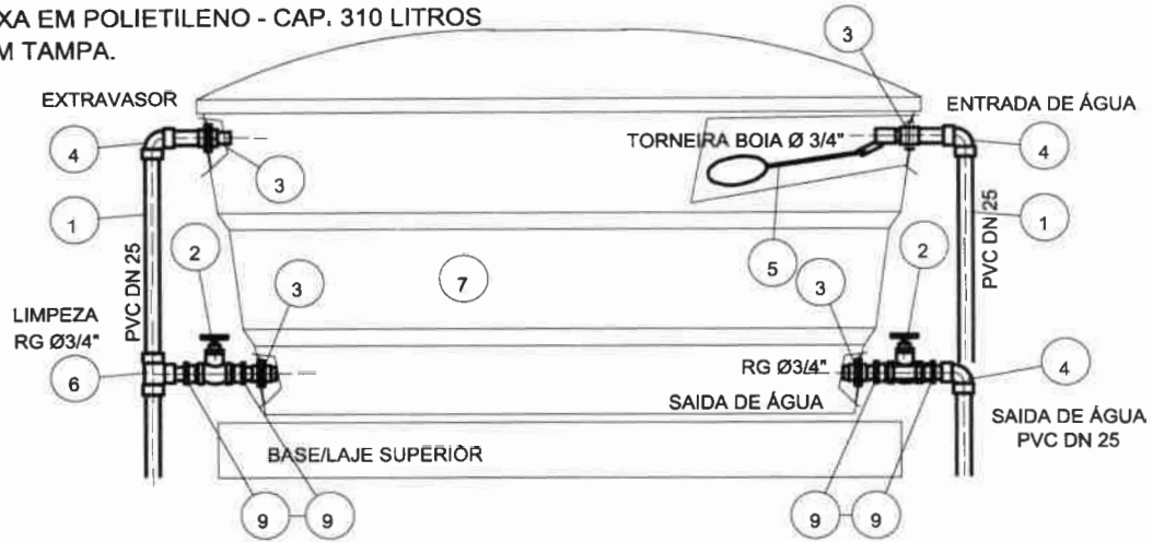
DETALHE - INSTALAÇÃO DA CAIXA D'ÁGUA. SEM ESCALA
