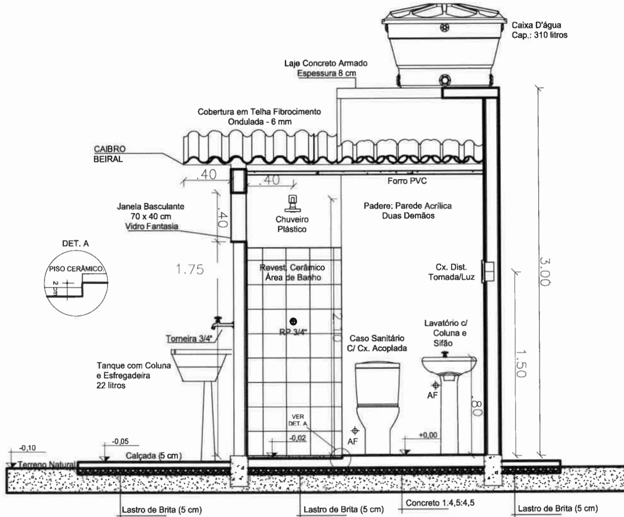
CORTE AA
