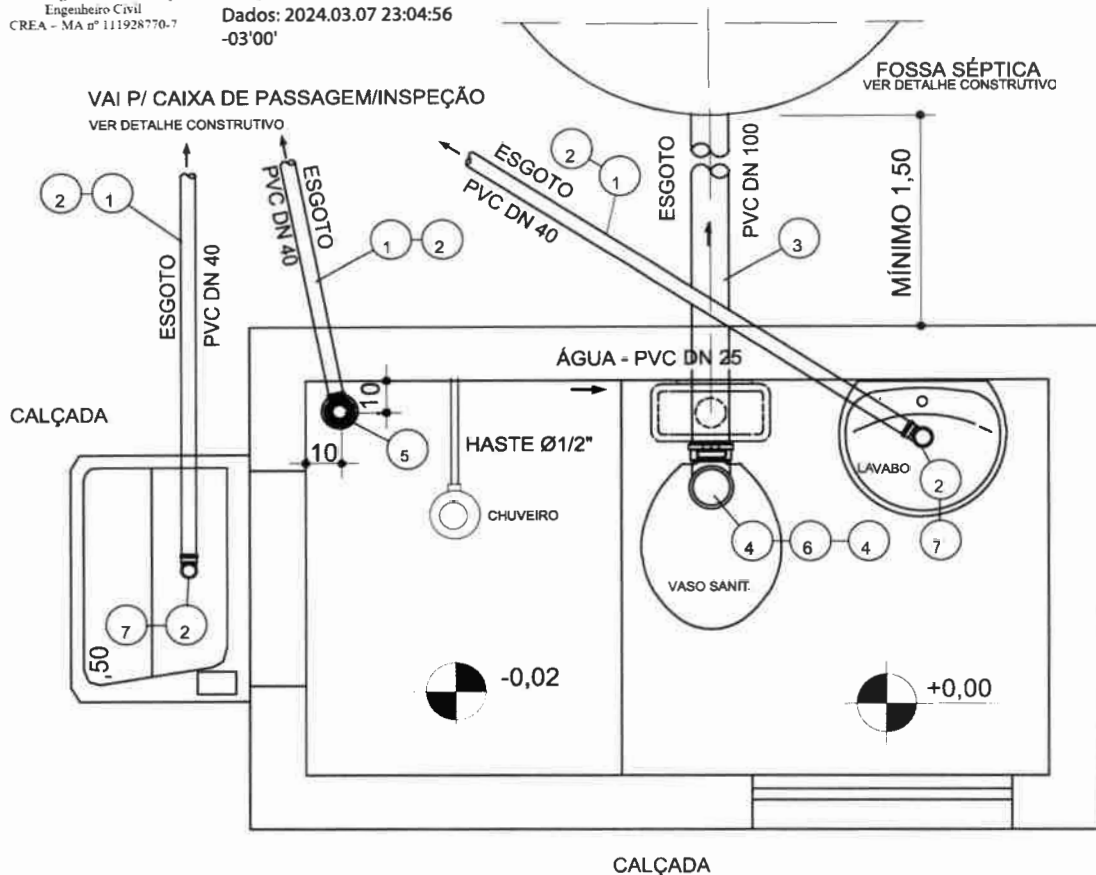
PLANTA - INSTALAÇÃO HIDROSSANITÁRIA
