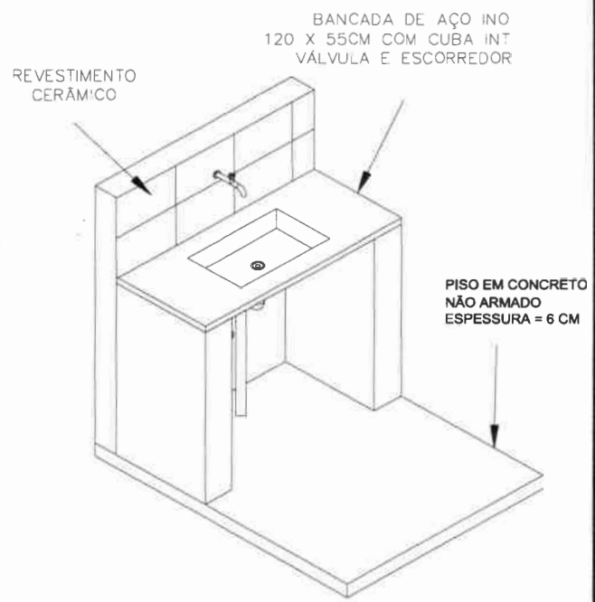
ISOMÉTRICO
