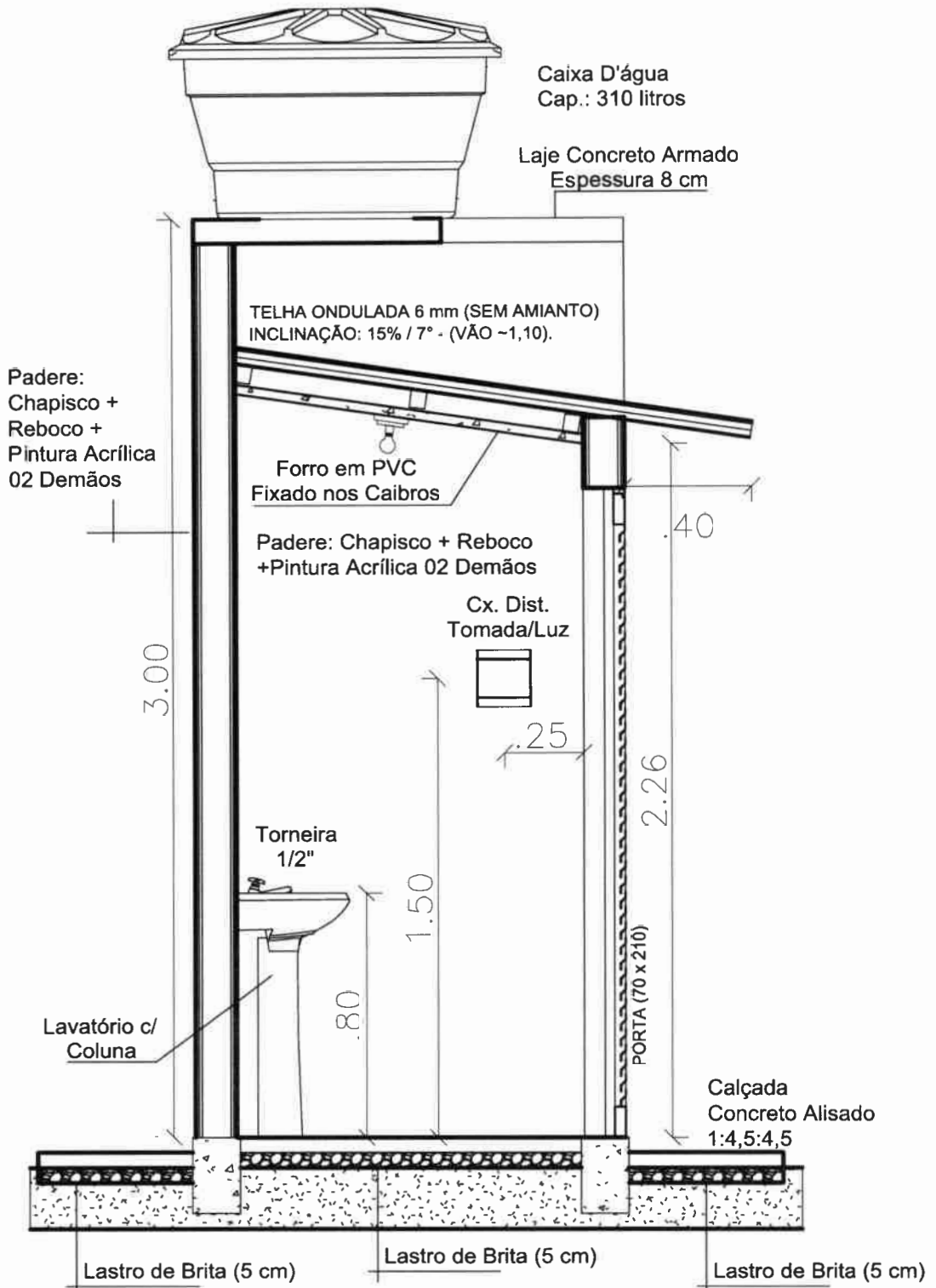
CORTE BB
