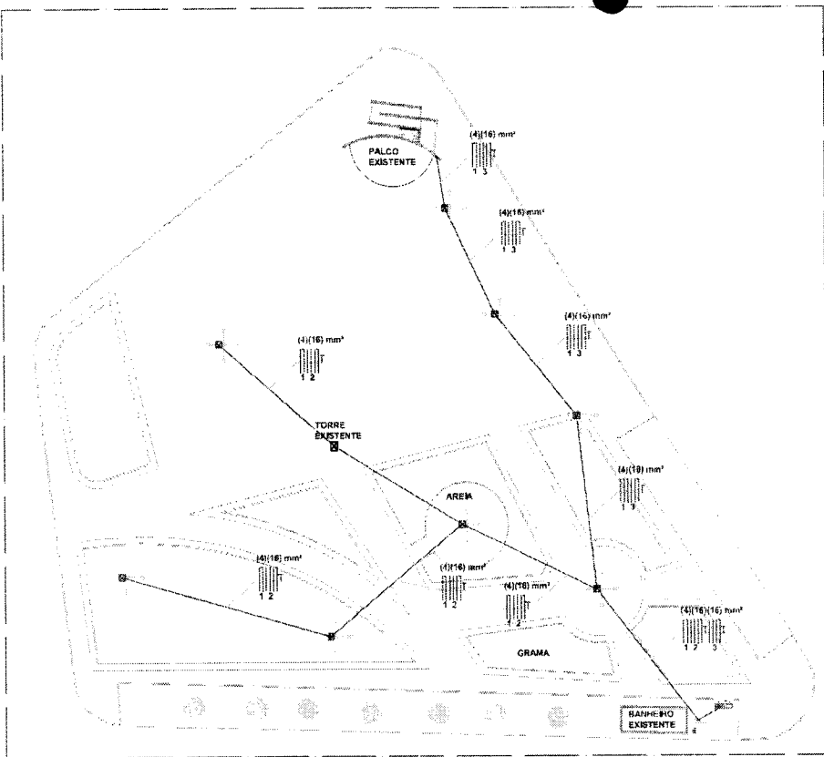
1 INSTALAÇÕES ELÉTRICAS
