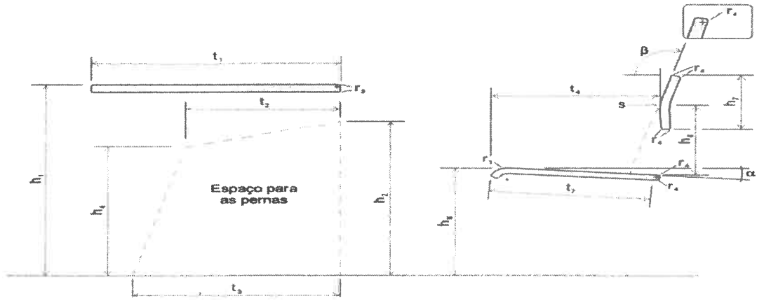
CORTE AA
