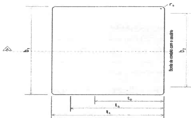
VISTA SUPERIOR
