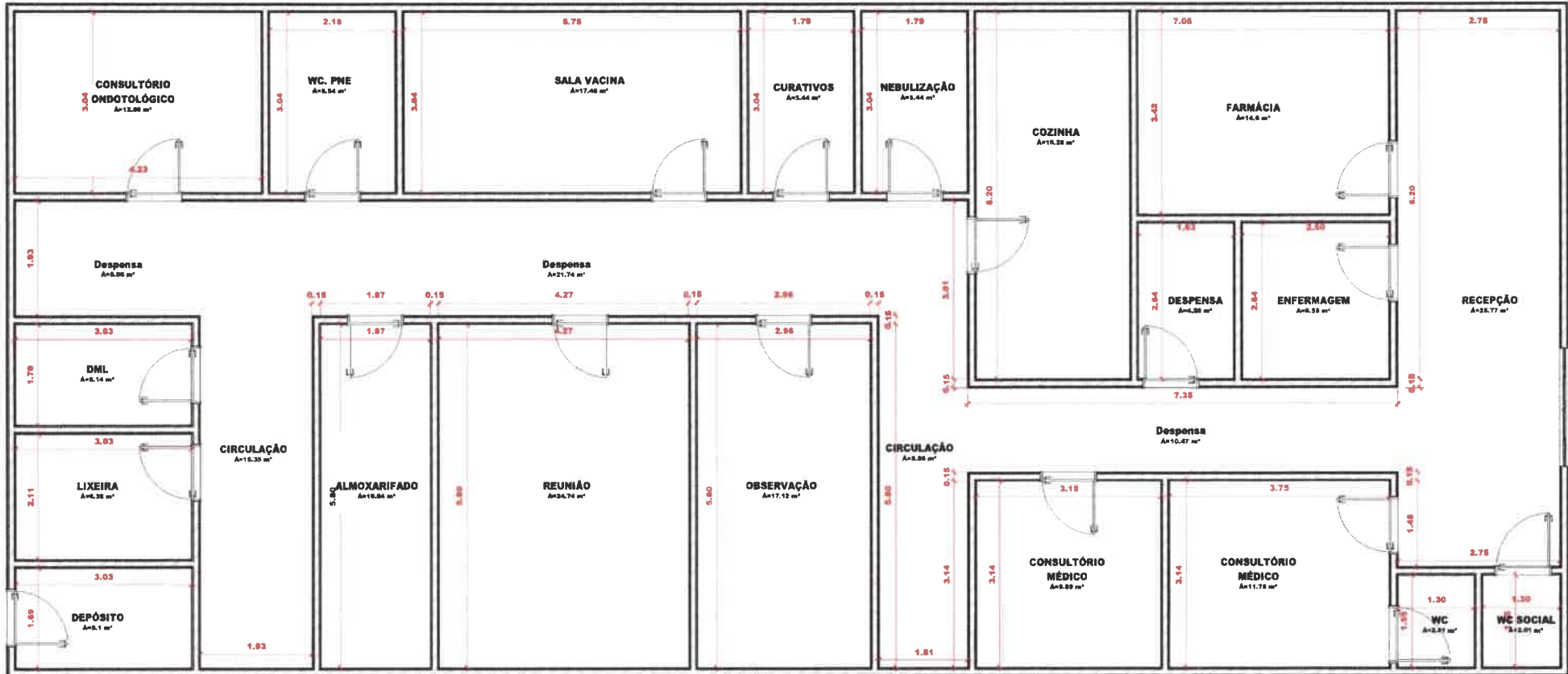
1 PLANTA BAIXA 1 : 50
