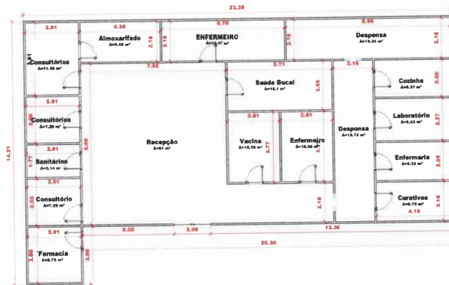
1 PLANTA BAIXA - UBS SEDE 1 : 100
