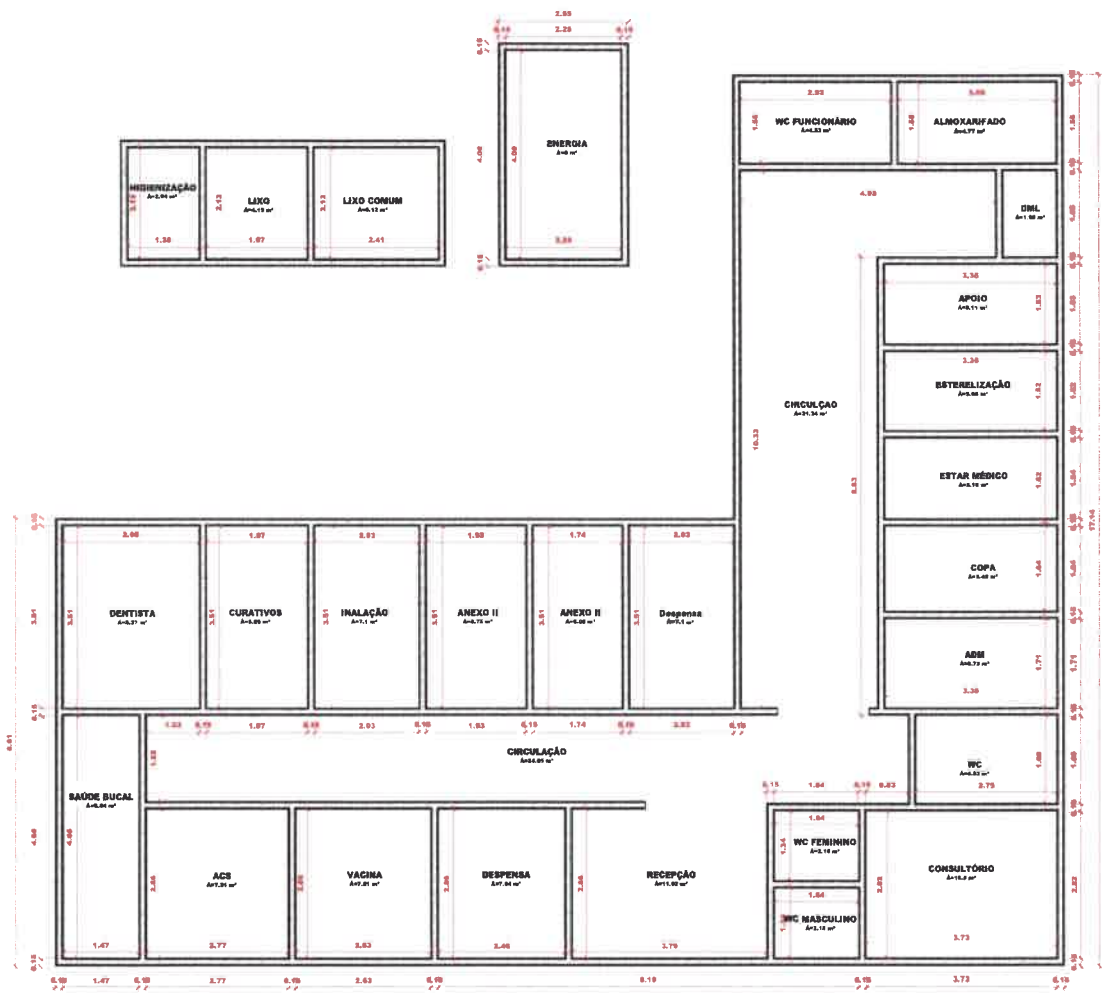
1 PLANTA BAIXA 1:50
